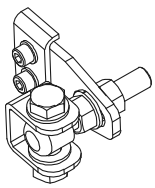
Set de charnières. Gonds réglables.
